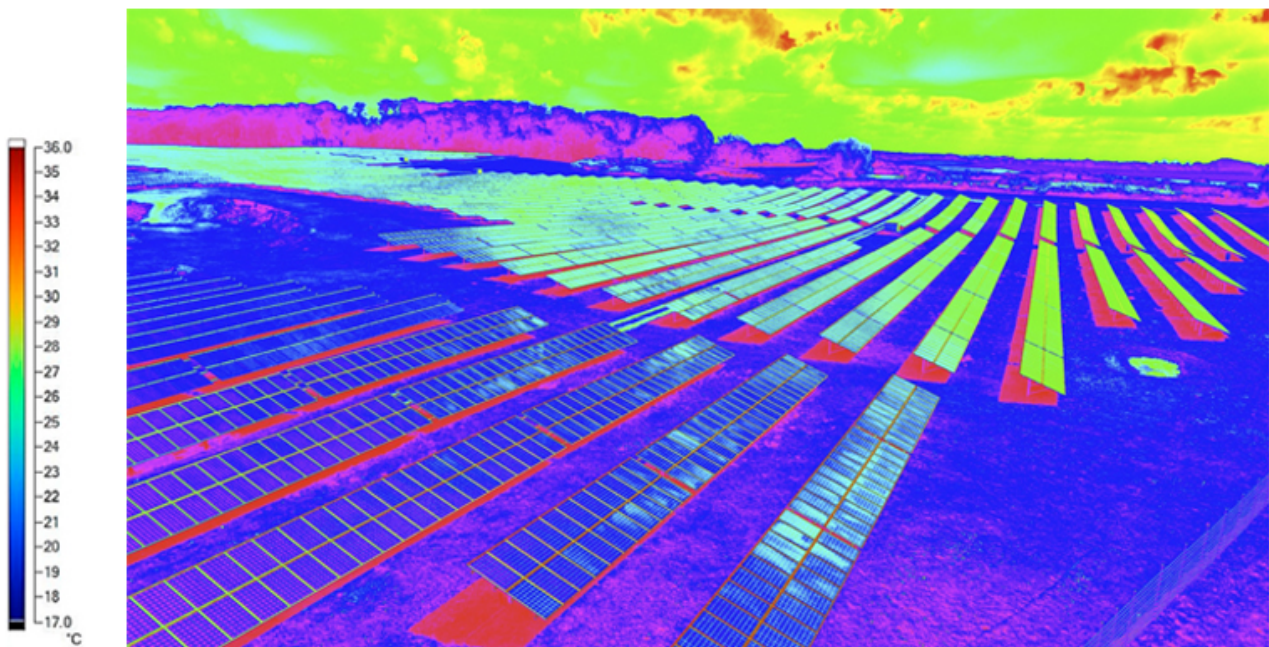
Esempio di termogramma su impianto fotovoltaico
